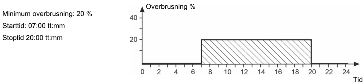
Figur 15: Overbrusning efter klokkeslæt
