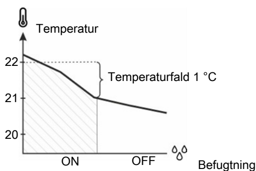
Figur 8: Faldende temperatur: Befugningen vil blive afbrudt hvis indetemperaturen er 1 °C under Indstillet temperatur. Befugningen vil ellers kunne få indetemperaturen til at falde yderligere.
