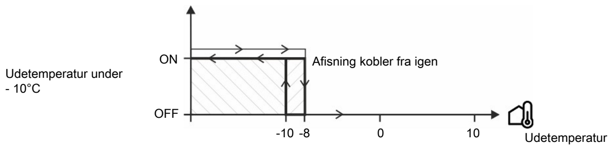
Figur 11: Aktivering af afisning
