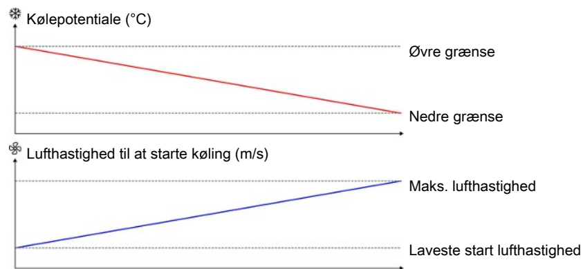
Figur 17: I områder med lav udefugt og et stort kølepotentiale, kan kølingen starte ved en lavere lufthastighed. Omvendt vil man i områder med lavt kølepotentiale vente så længe som muligt med at starte kølingen, så den starter ved maksimum lufthastighed.
