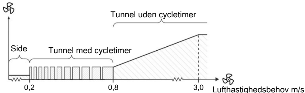
Figur 12: Ventilationsforløb med cycletimer ved tunnel-ventilation
