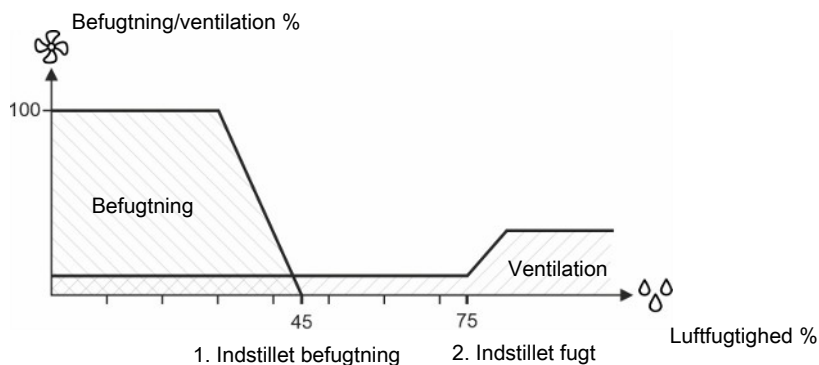
Figur 7: 1. Faldende luftfugtighed. Luftfugtigheden er under Indstillet befugning. Staldcomputeren starter befugningen. 2. Stigende luftfugtighed. Luftfugtigheden er over Indstillet fugt. Staldcomputeren øger ventilationen.
