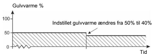
Figur 23: Gulvvarme uden temperaturføler
